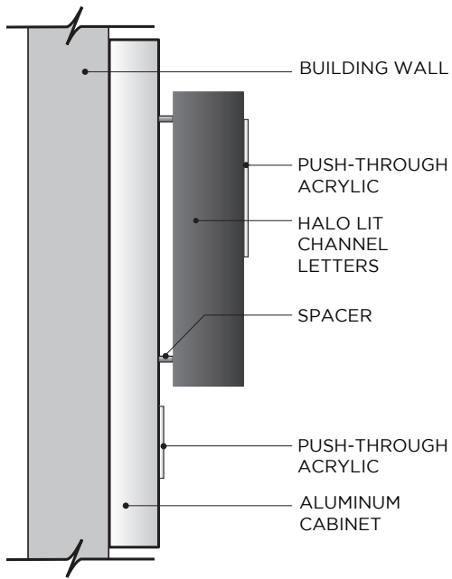
4 Side view N.T.S.
